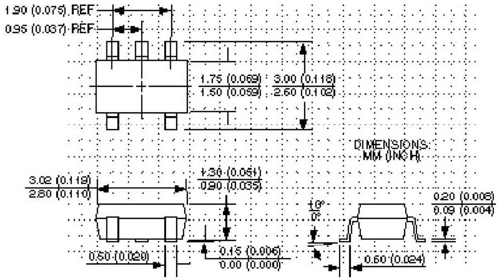
SOT-23-5 (M5)
